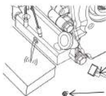
ORIFICE / COUVERCLE DE REMPLISSAGE DE L'HUILE
